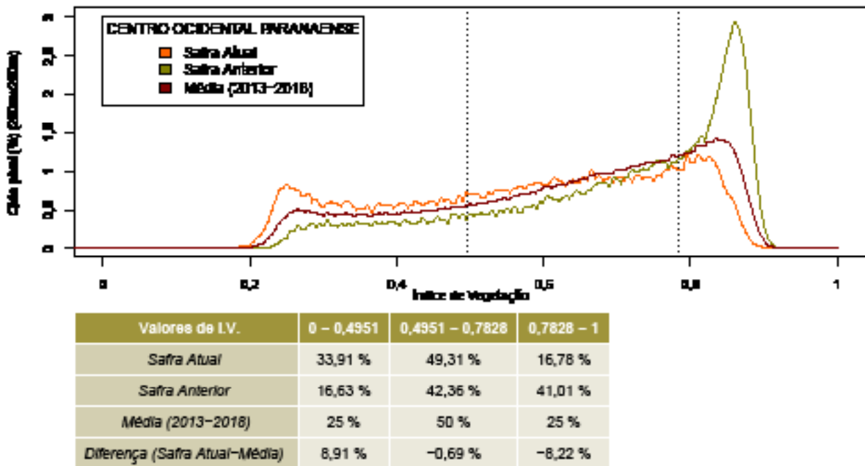
Gráfico 31 - Quantificação de áreas em razão do IV (histogramas) - Centro Ocidental Paranaense
