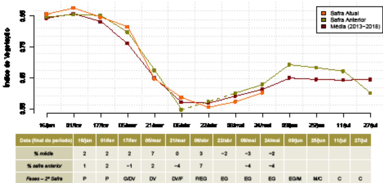
Gráfico 42 - Evolução temporal do IV - Centro Sul Paranaense
