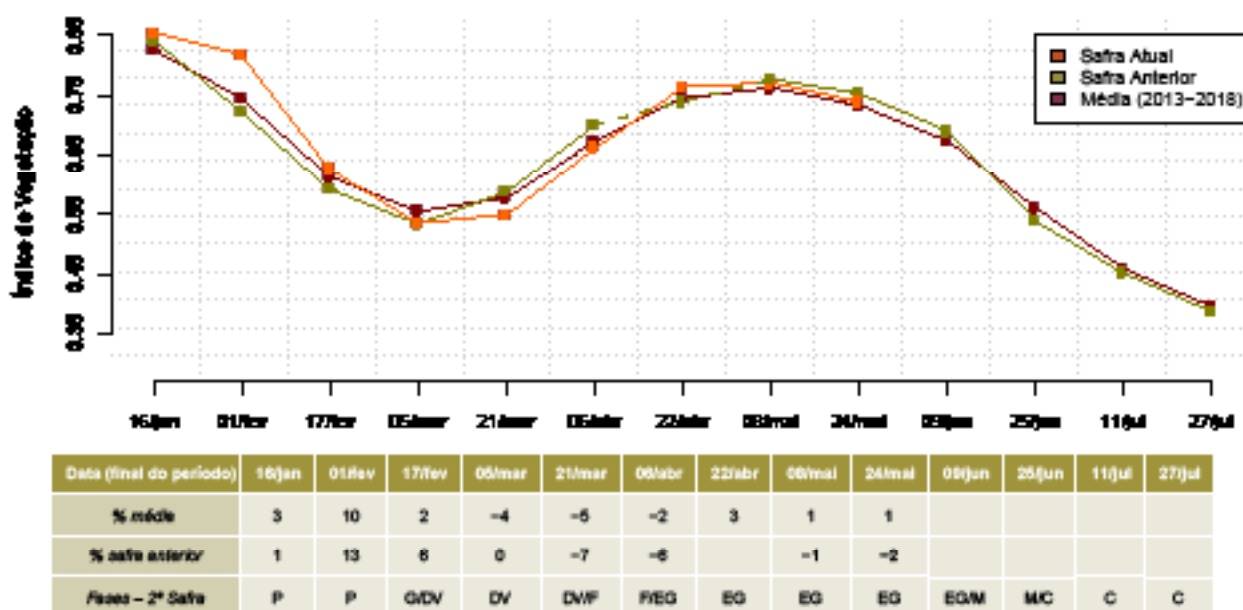
Gráfico 22 - Evolução temporal do IV - Sul Goiano
