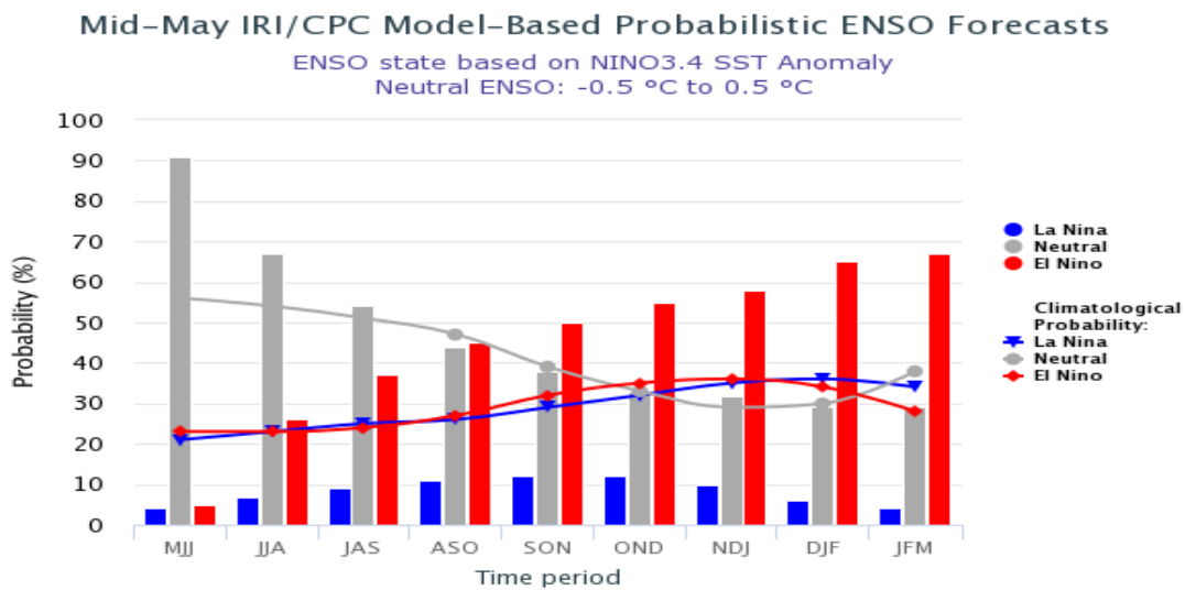
Gráfico 2 - Previsão probabilística do IRI para ocorrência de El Niño ou La Niña
