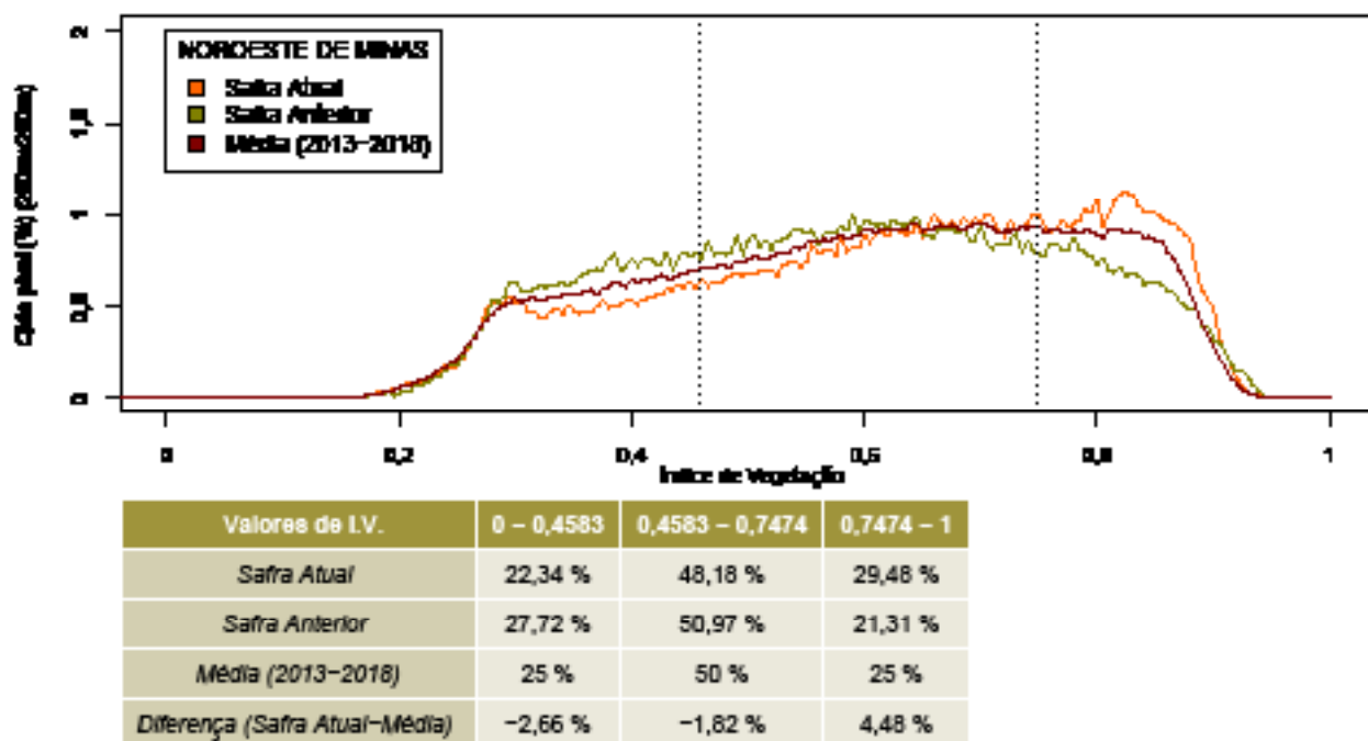
Gráfico 23 - Quantificação de áreas em razão do IV (histogramas) - Noroeste de Minas
