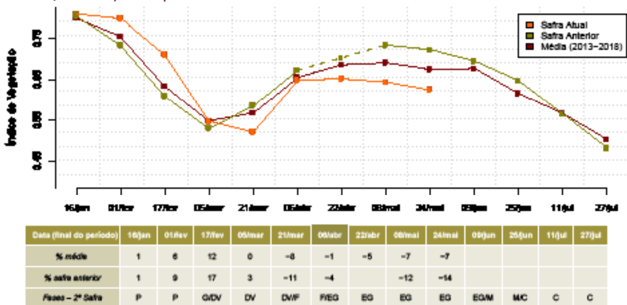
Gráfico 41 - Evolução temporal do IV - Noroeste Paranaense
